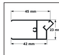
Profilo calamita
