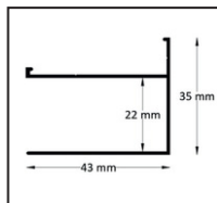
Profilo muro
