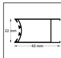
Profilo cerniera
