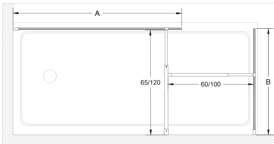
Profilo muro
