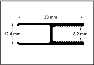
Profilo vetro
