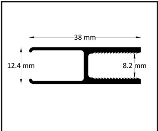
Profilo vetro
