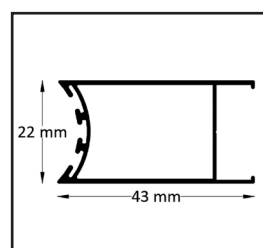
Profilo cerniera
